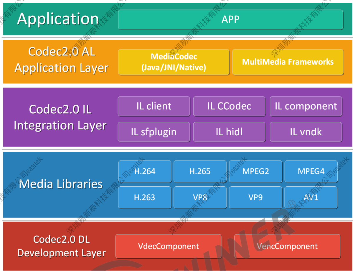
图 10-1: Codec2 架构图
