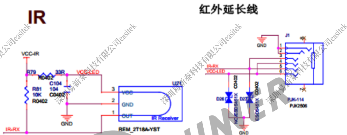
图 2-1: IR-RX 模块
