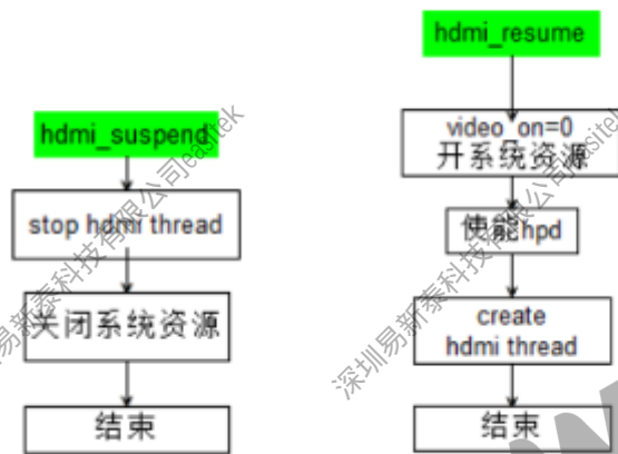
图 6-9: 休眠唤醒
