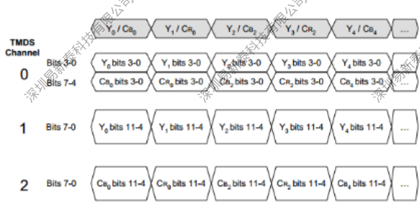
图 6-5: 422 打包格式
