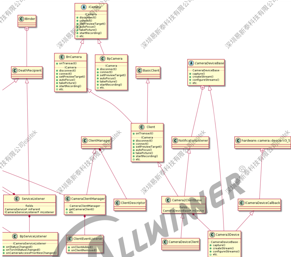
图 4-3: CameraService 类图
