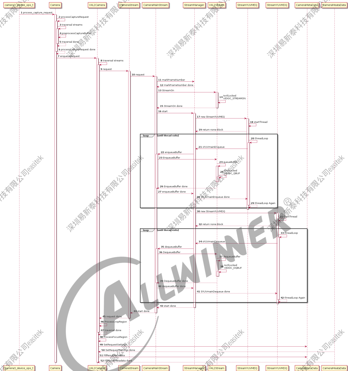
图 5-7: process_capture_request
